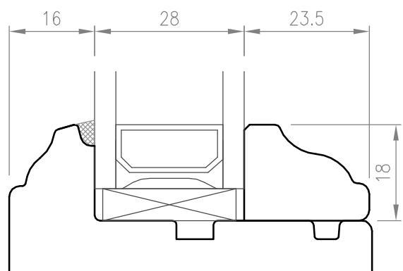
Fermavetro Tipo 3
